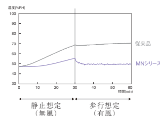
④靴内湿度・側面
