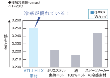
図③ 着たときすぐの快適性
