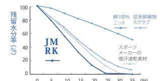
3.速乾性データ
