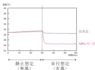
①靴内温度・土踏まず部分
