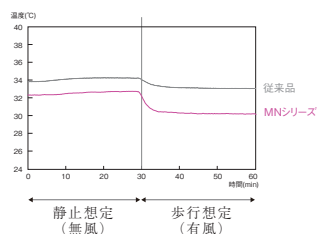
③靴内温度・側面
